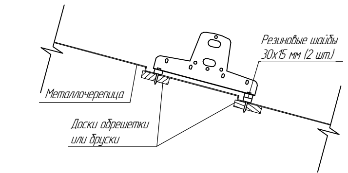
Схема крепления на металлочерепицу
