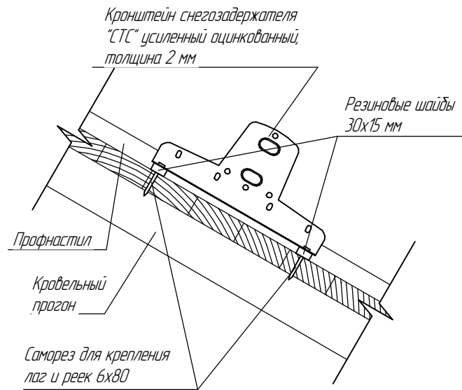
Узел крепления на кровлю из профлиста
