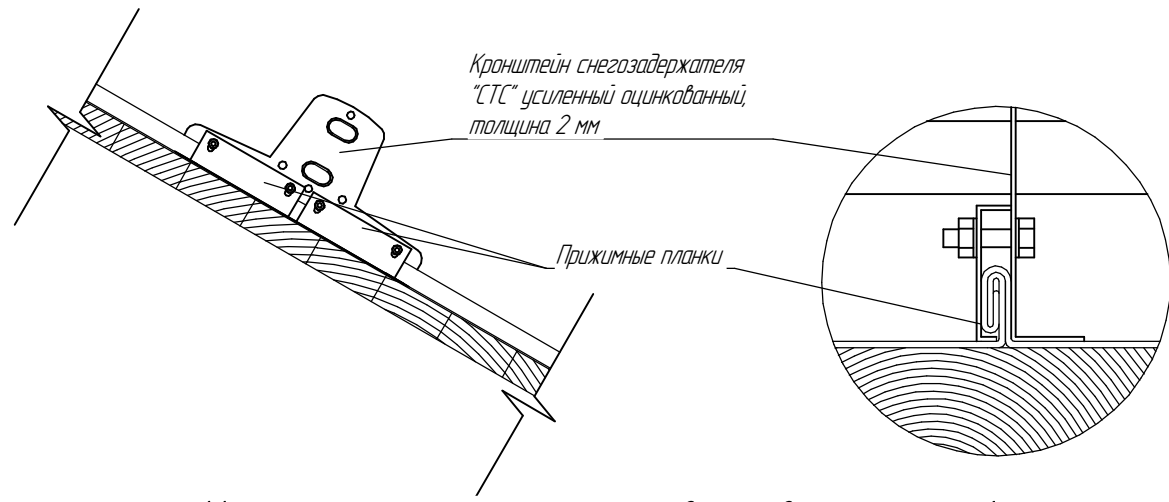
Узел крепления на фальцевую кровлю тип 1
