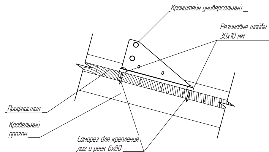
Узел крепления на кровлю из профлиста
