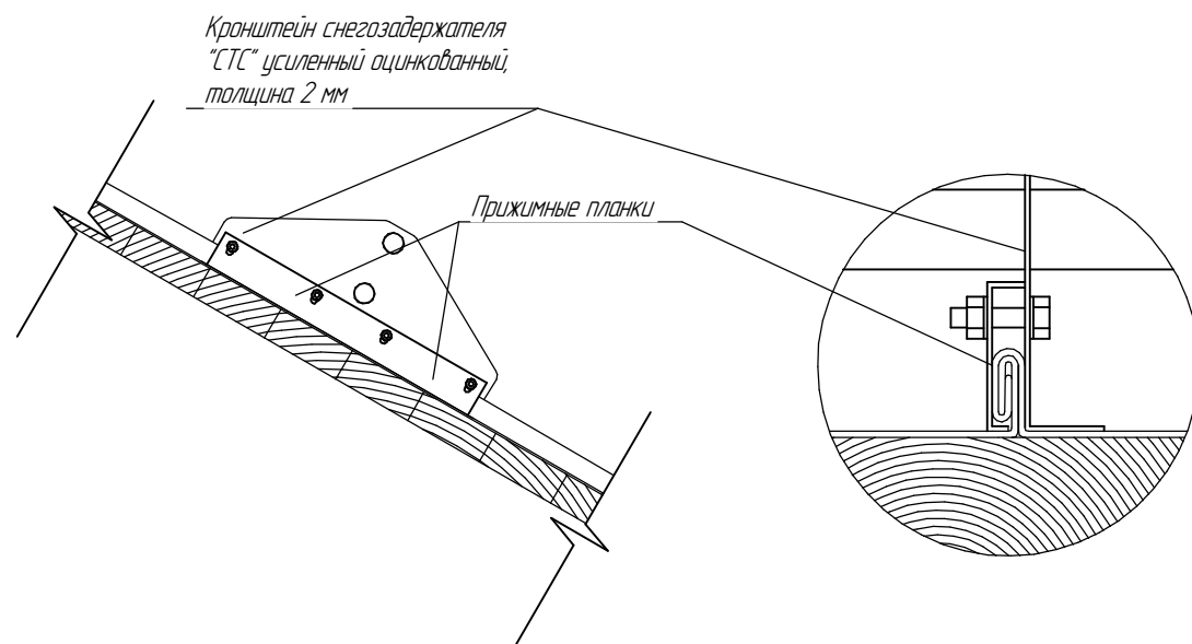
Узел крепления на фальцевую кровлю тип 1
