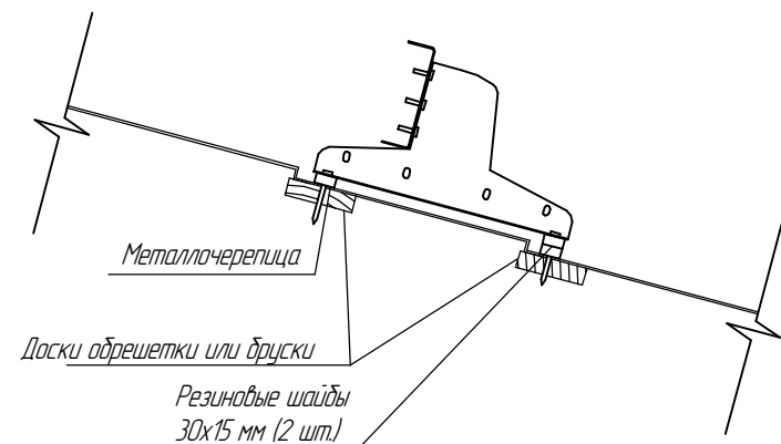
Схема крепления на металлочерепицу
