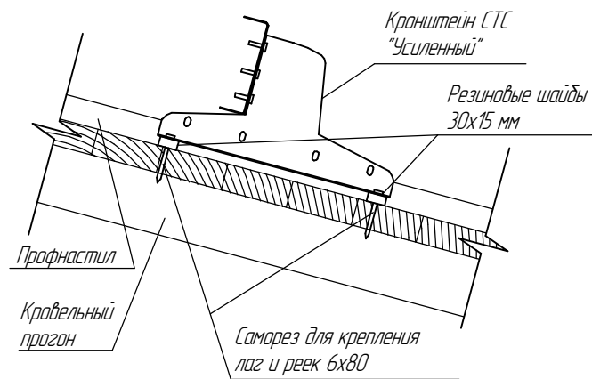
Узел крепления на кровлю из профлиста
