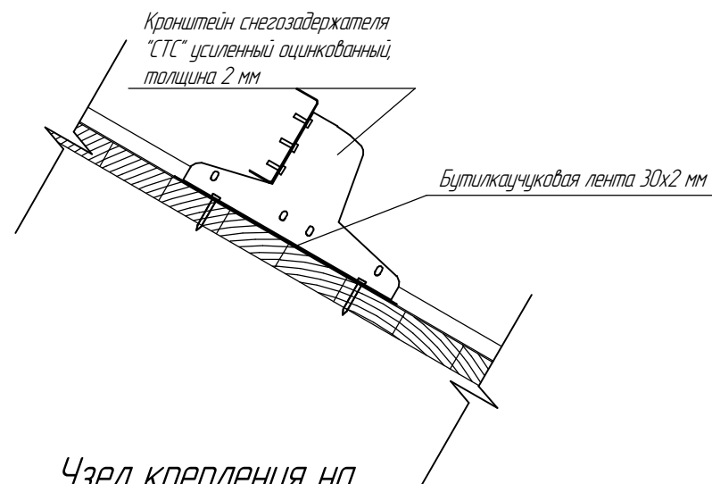
Узел крепления на кровлю из профлиста
