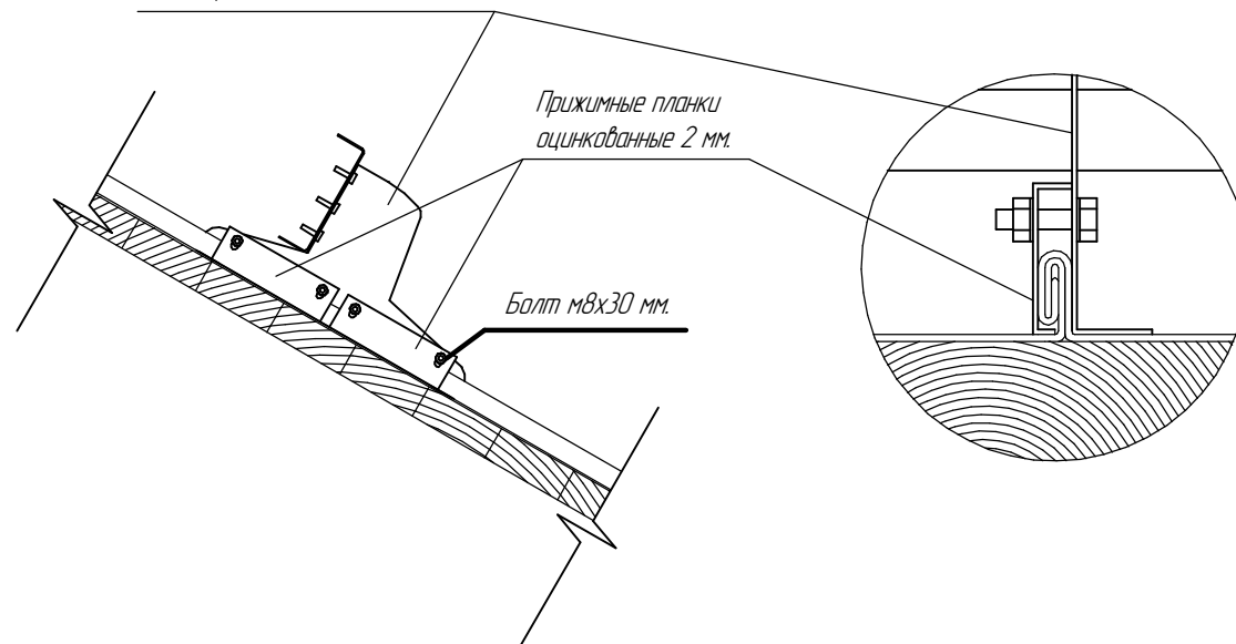
Узел крепления на фальцевую кровлю тип 1
