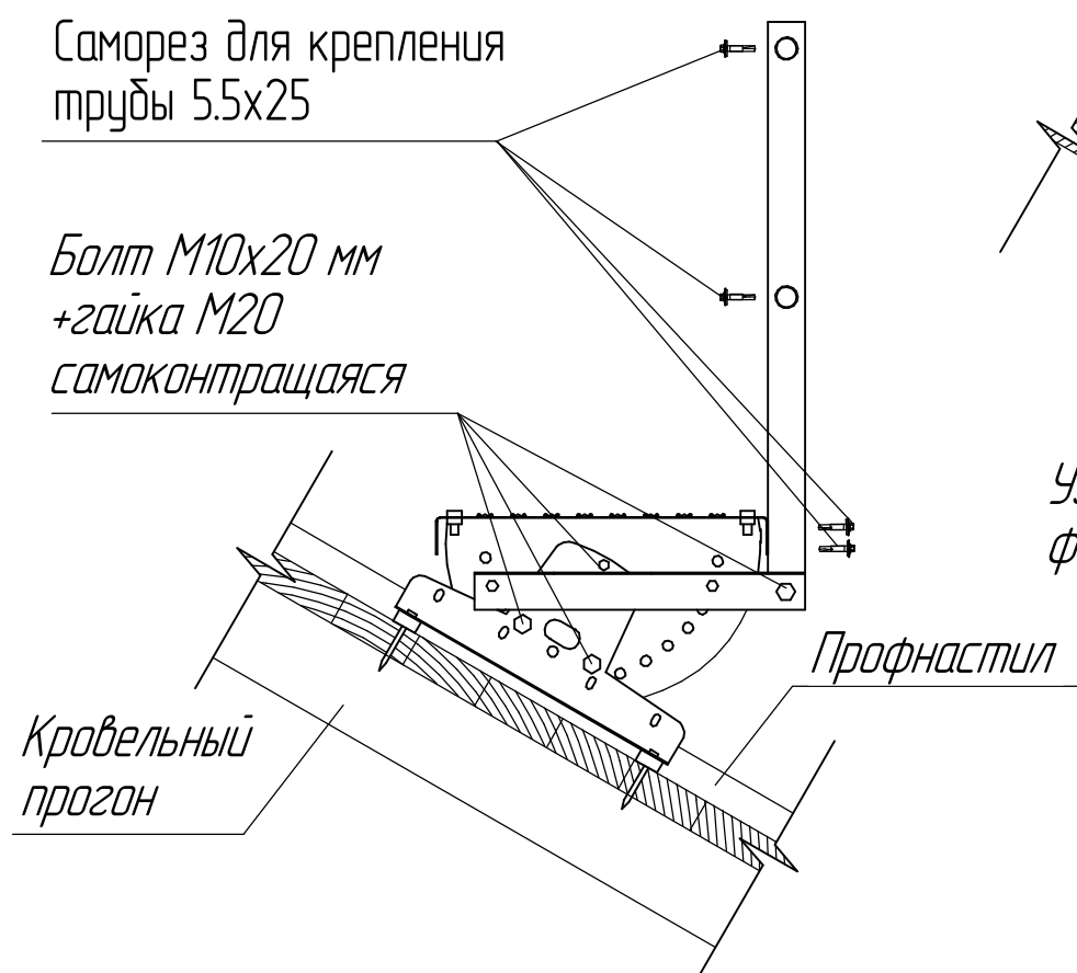
Узел крепления на кровлю из профлиста
