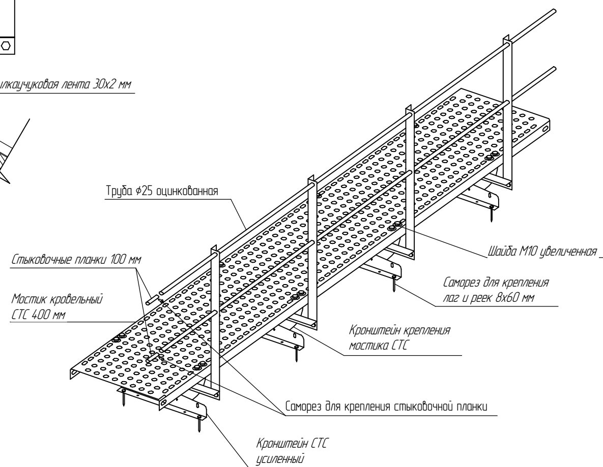
Узел крепления на фальцевую кровлю тип 2
