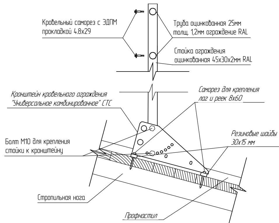
Узел крепления на кровлю из профлиста
