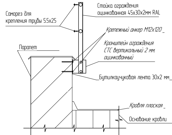
Узел крепления на парапет
