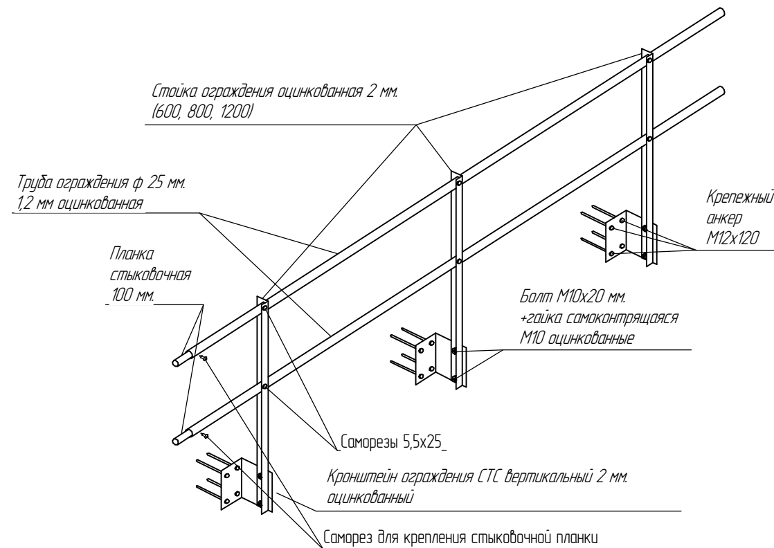
Узел крепления на парапет
