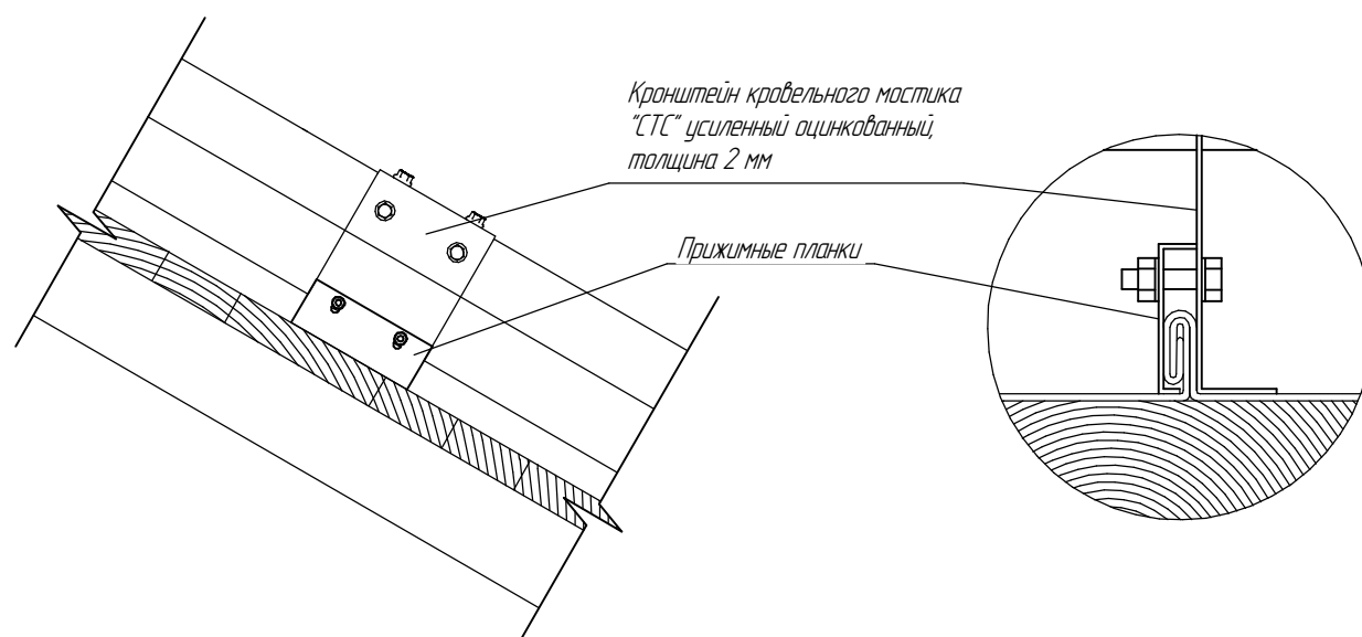
Узел крепления на фальцевую кровлю
