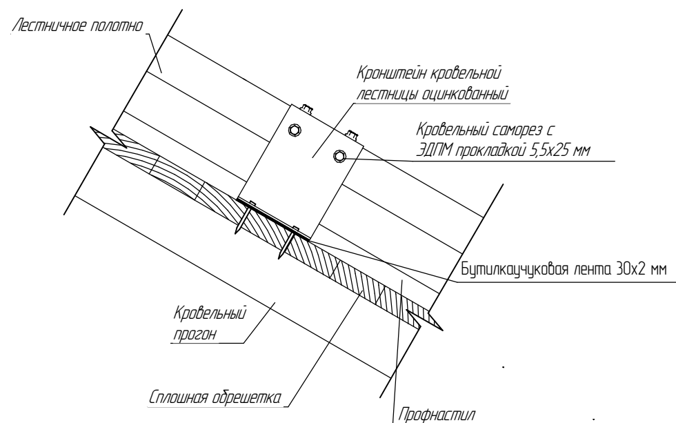
Узел крепления на кровлю из профлиста
